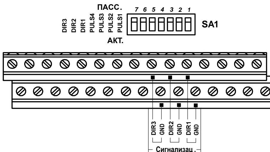
Рис.26. Маркировка коммутационных элементов подключения входов «Сигнализац.».
