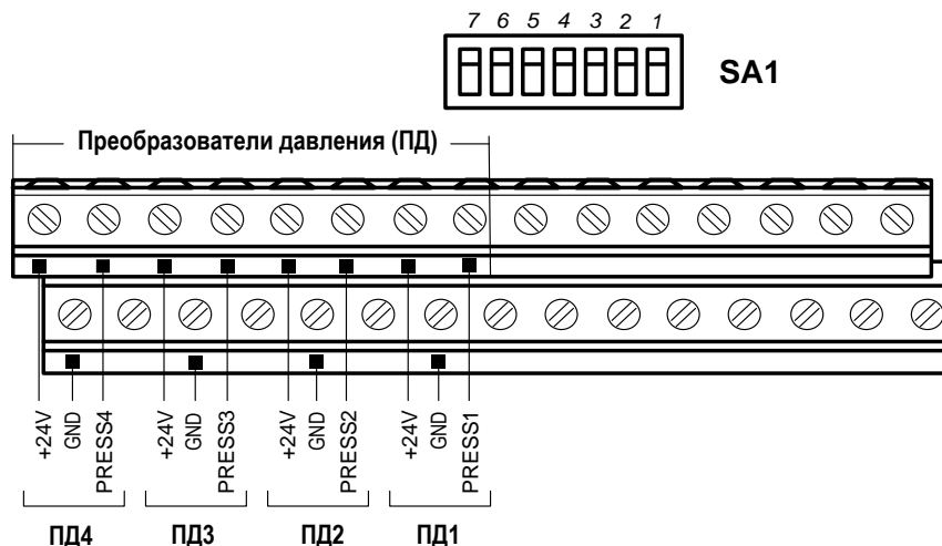
Рис.30. Обозначение коммутационных элементов подключения ПД.
